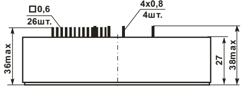
Рисунок 8.4 – Габаритные размеры М31-5,10-1,2,6А2*
