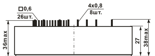
Рисунок 8.3 – Габаритные размеры М31-5,10-1,2,6А3*
