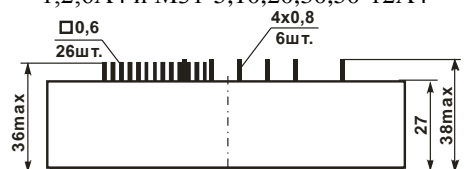
Рисунок 8.2 – Габаритные размеры М31-20,30,50,70,100-1,2,6А4 и М31-5,10,20,30,50-12А4*
