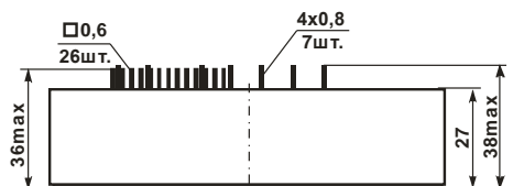
Рисунок 8.1 – Габаритные размеры М31-5,10-1,2,6А4*
